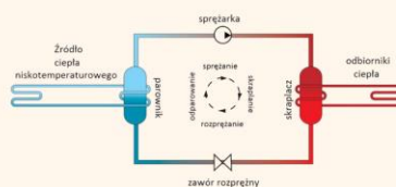
Schemat działania pompy ciepła
