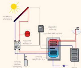
Schemat instalacji kolektorów słonecznych ( www.budujemydom.pl )
